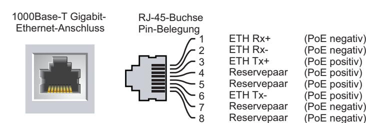
Abbildung 5 Pin-Belegung des Gigabit-Ethernet-Anschlusses
